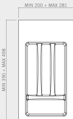
Cutlery trays height / Altezza portaposate 45 mm
